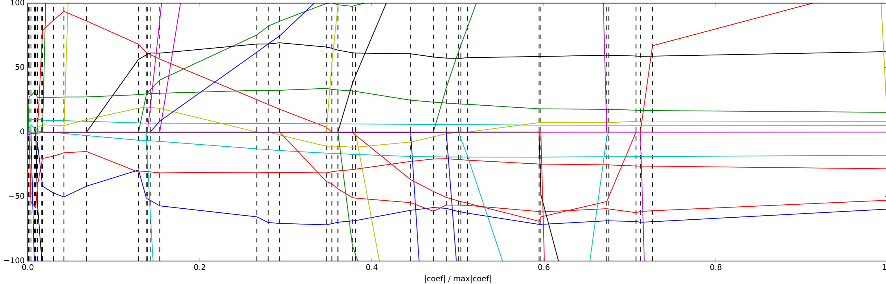
LASSO Path
