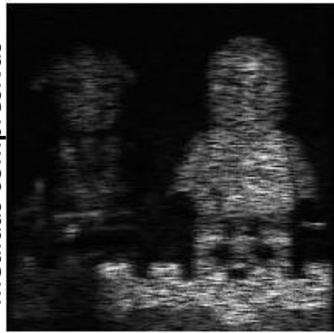
PSNR 29.7756
