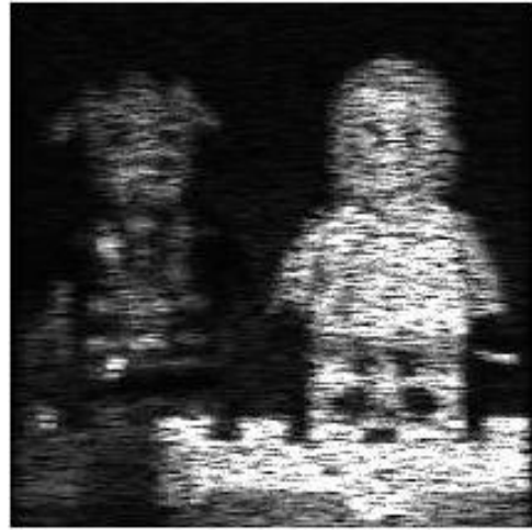
PSNR 19.3972
