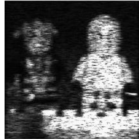
PSNR 15.7227
