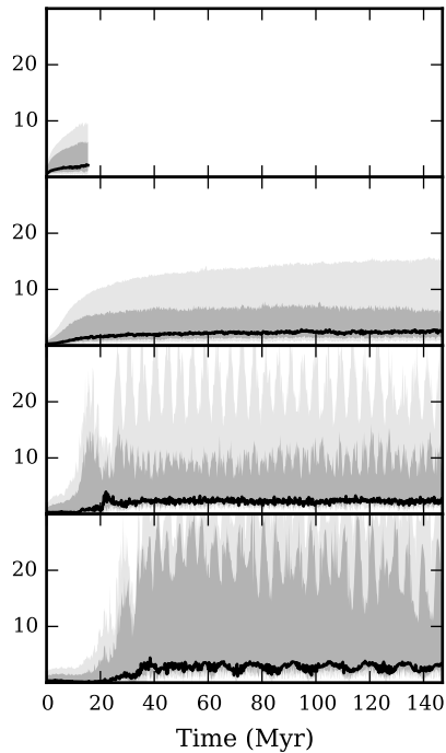
Inclination (Deg)
