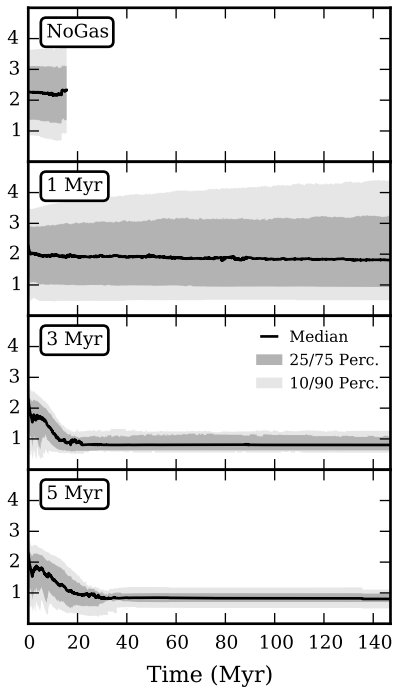
Semi-Major Axis (AU)
