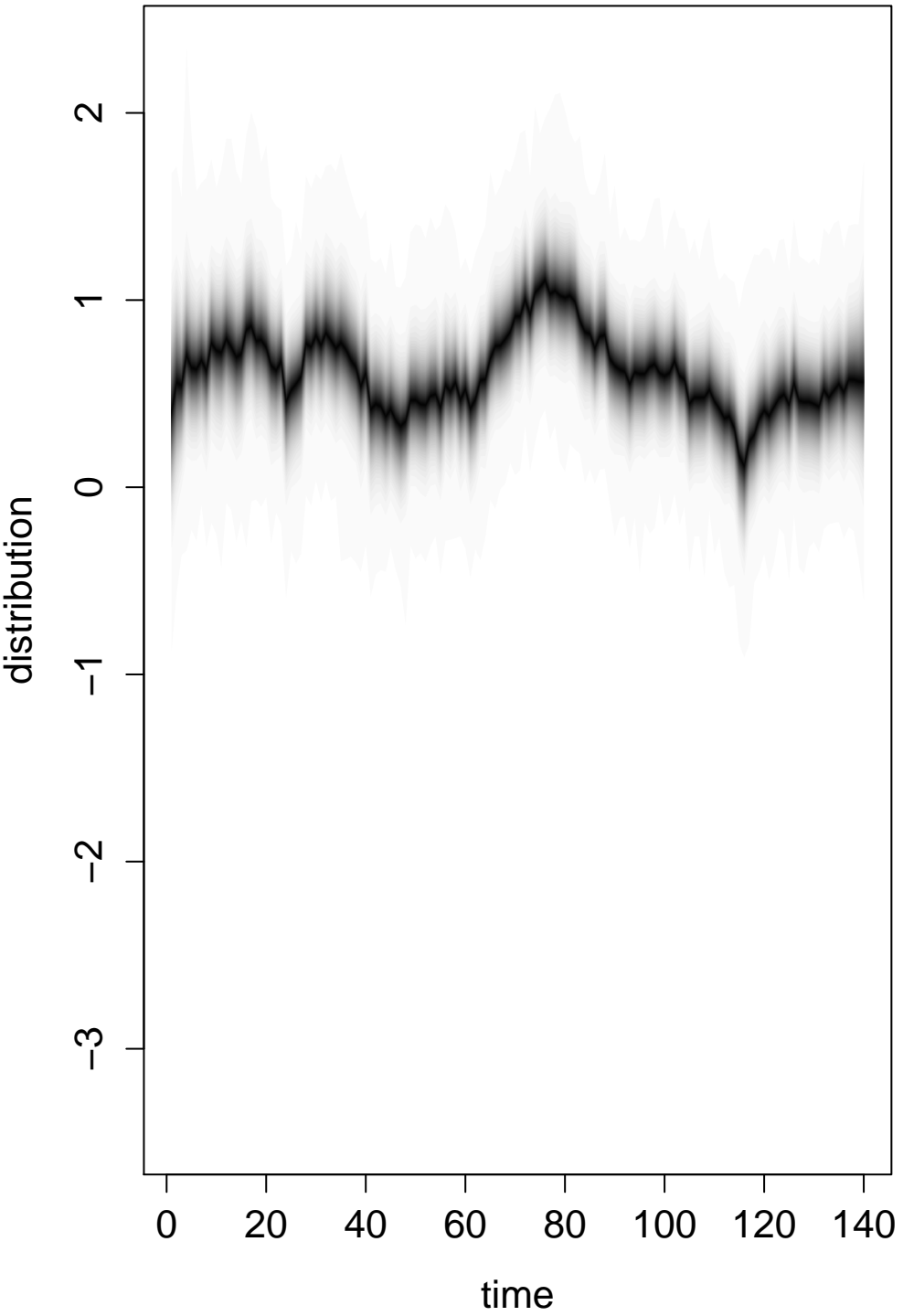
trend
