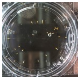
SMOW
