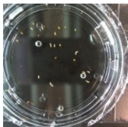
5% D2O
